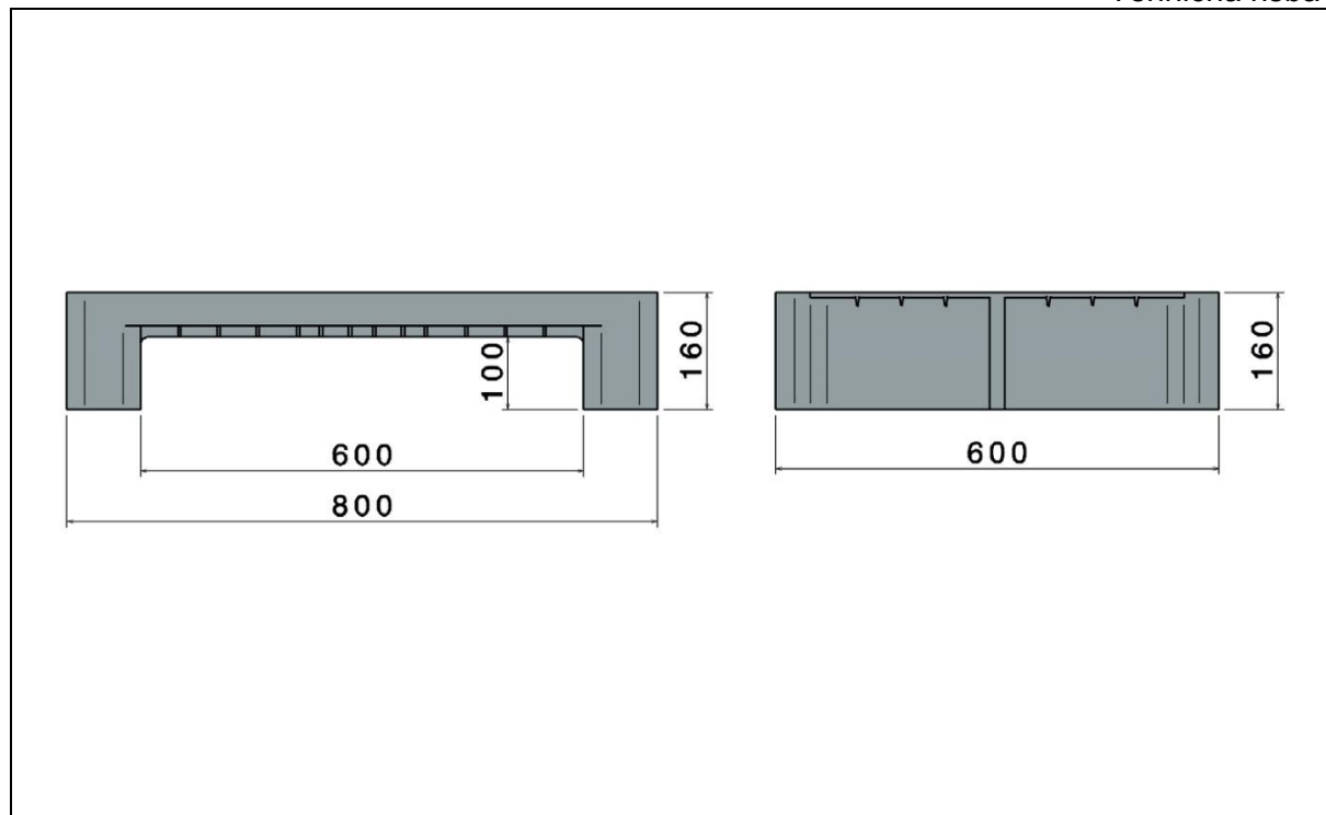
Tehnična risba
